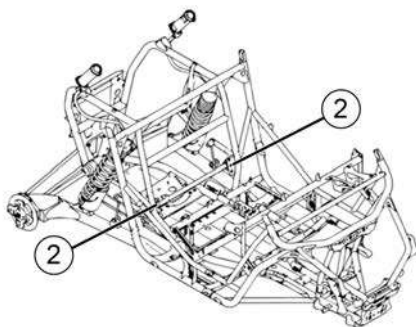
② Buchas da haste estabilizadora traseira (uma em cada lado do veículo)
